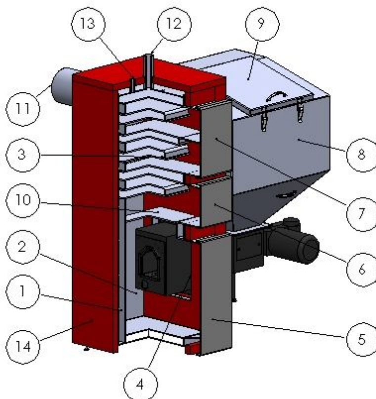
Rys.1. Kocioł "Technix (ECONOMY)"
