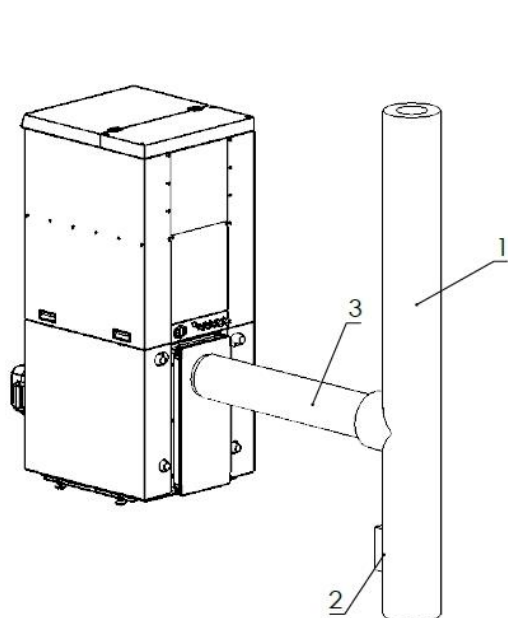
Rysunek 14 - Podłączenie do instalacji kominowej – proste 1 – Przewód kominowy; 2 – Wyczystka kominą; 3 – Zaizolowane podłączenie do kominą
