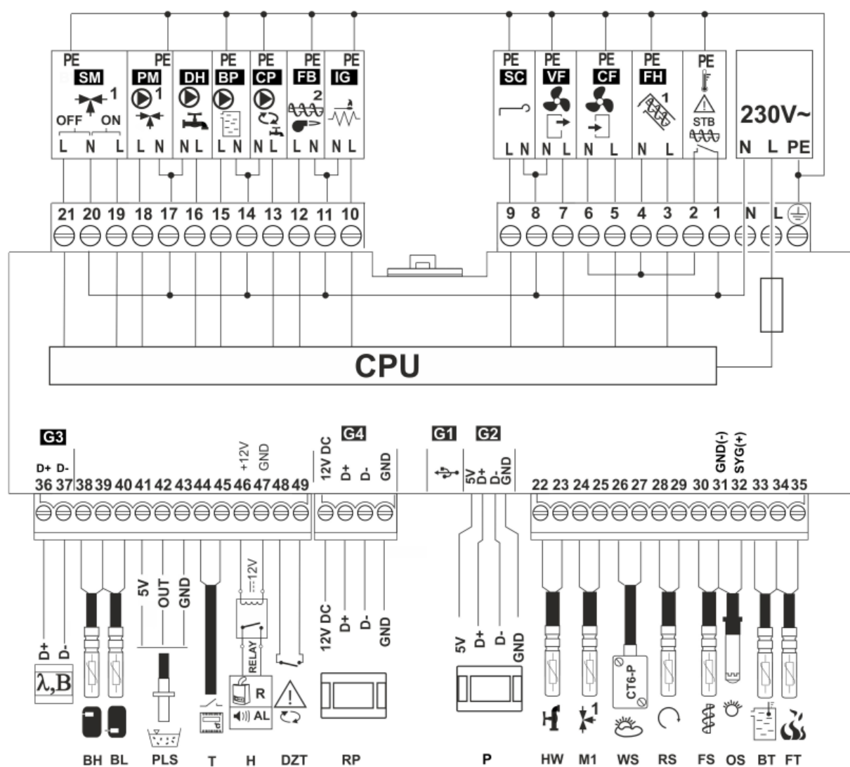
Osprzęt kotła należy podłączyć zgodnie z poniższym schematem do sterownika ecoTOUCH860-P3-C:
