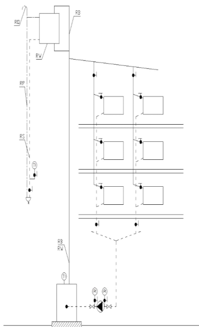
Rysunek 1b Schemat zabezpieczenia instalacji ogrzewania wodnego, wyposażonej w jeden kocioł lub wymiennik ciepła, rozdział górny, pompa zamontowana na powrocie wg PN-91/B-02413
